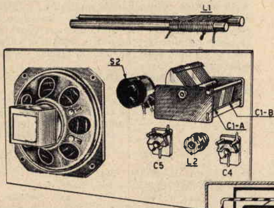
Fig. 5 - Disposizione componenti principali su telaio in faesite o altro materiale isolante.
